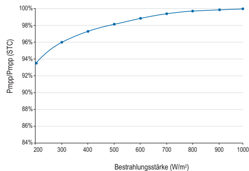
Einfluss der Bestrahlungsstärke auf den PmpP — Mittelwert Siliken-Module
