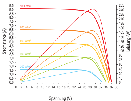
SLK60M6L - 240 Wp I-U und Pmax-Kurven bei unterschiedlichen Bestrahlungsstärken bei 25°C
