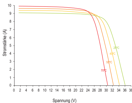
SLK60M6L - 240 Wp I-U-Kurven bei unterschiedlichen Zellentemperaturen bei 1000 W/m²
