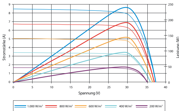
Stromspannungs- & Leistungs-Spannungskennlinie (220-20)
